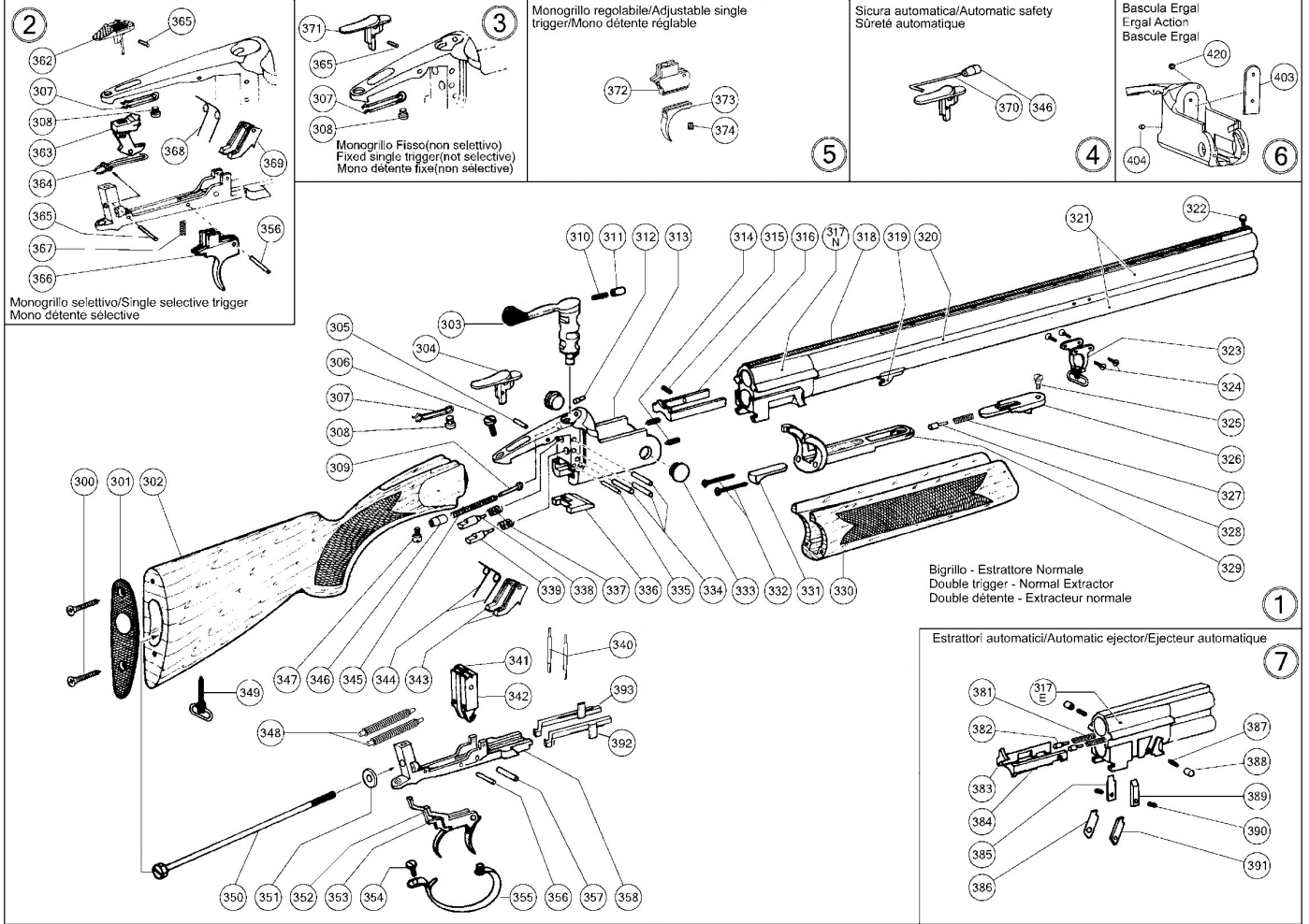
ESPLOSO FUCILE SOVRAPPONTO - OVER/UNDER EXPLODED-VIEW - ÉCLATÉ FUSIL SUPERPOSÉ
